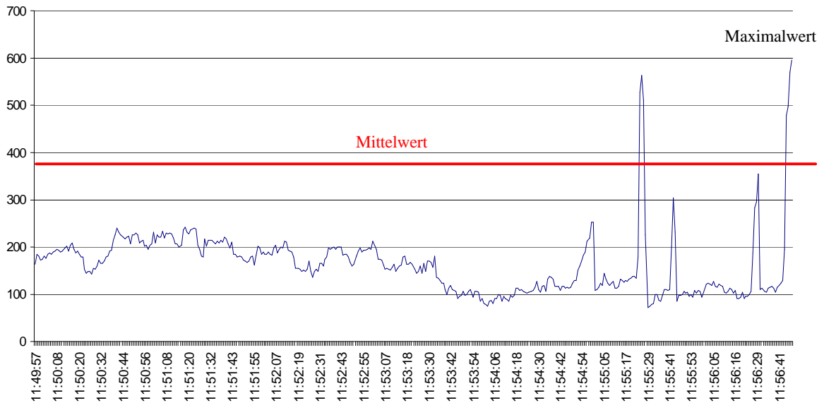
Abb. 6 Zeitlicher Verlauf der magnetischen Flussdichte in nT an MP-1 (lineare Skalierung)
