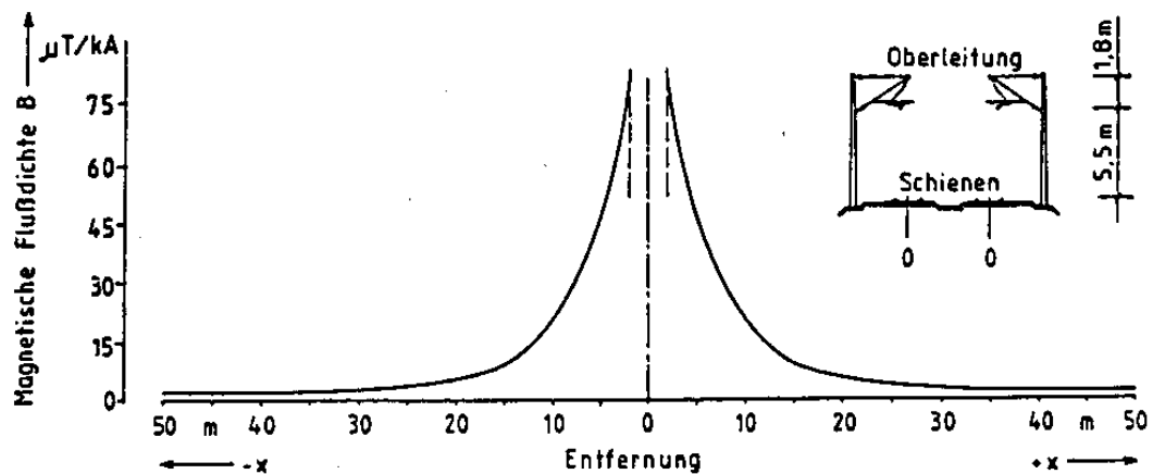
Abb.2 Theoretischer Verlauf der maximalen magnetischen Flussdichte je 1000 A Fahrstrom im Bereich einer zweigleisigen Bahnstrecke mit Wechselstromoberleitung Quelle: DIN VDE 0228 Teil 6
