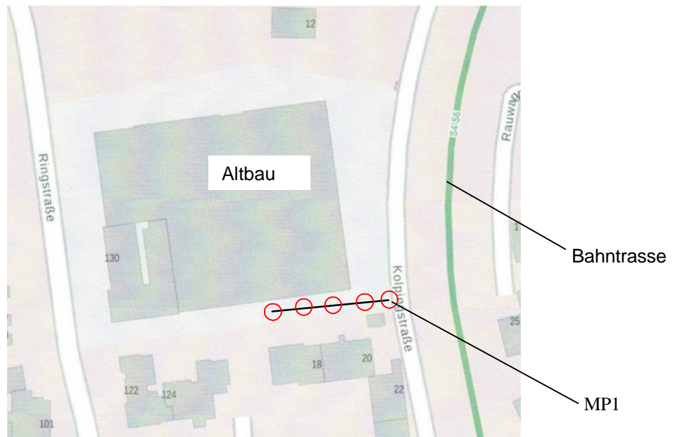
Abb. 1.1 Lage der Messachse in Horizontalebene
