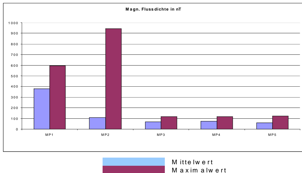
Abb. 7 Verlauf der mittleren und maximalen magnetischen Flussdichte [nT] in Abhängigkeit der Entfernung vom Gleiskörper
