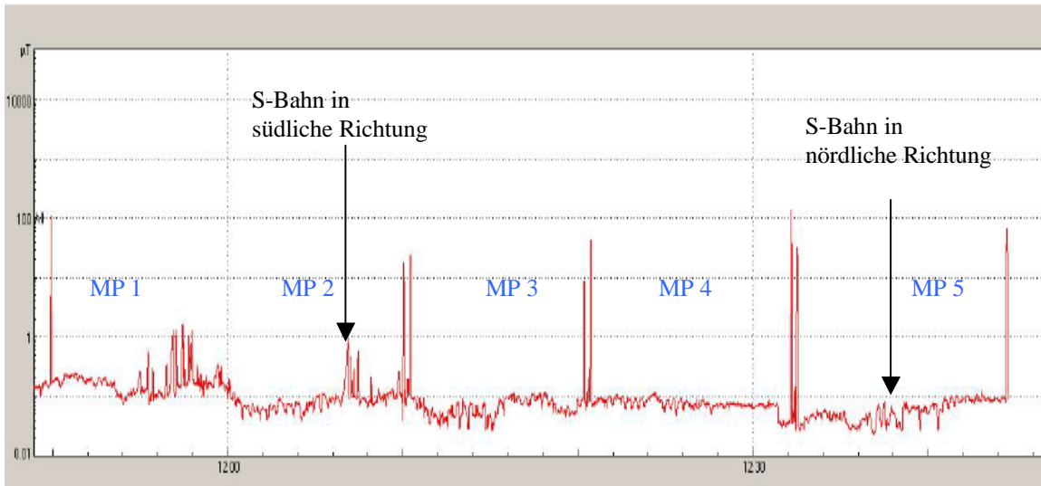
Abb. 5 Zeitgleicher Gesamtverlauf der magnetischen Flussdichte in \mu\text{T} (logarithmische Skalierung der Messwerte)
