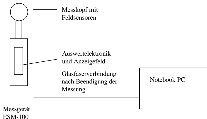
Abb.3 verwendetes Messgerät
