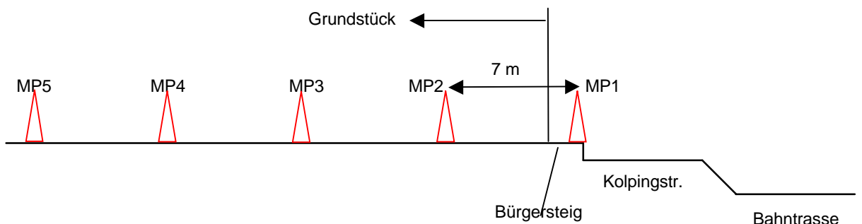
Abb. 1.2 Messpositionen in Vertikalebene (nicht maßstabsgerecht)
